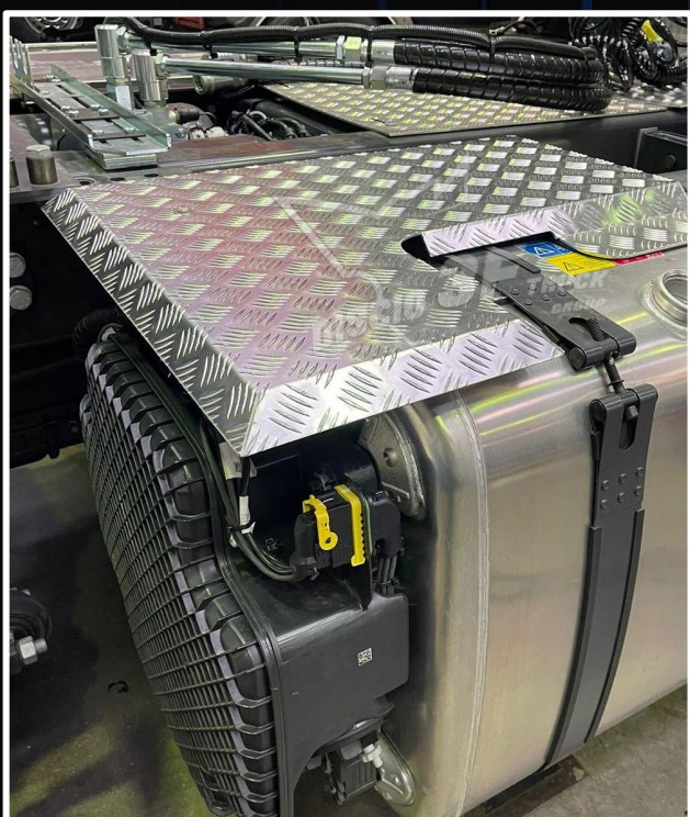
3F155SC.S LAMIERA PROTEZIONE UNITA' DI OTTIMIZZAZIONE CARBURANTE – FOU FUEL SCANIA N/G - LATO DX
